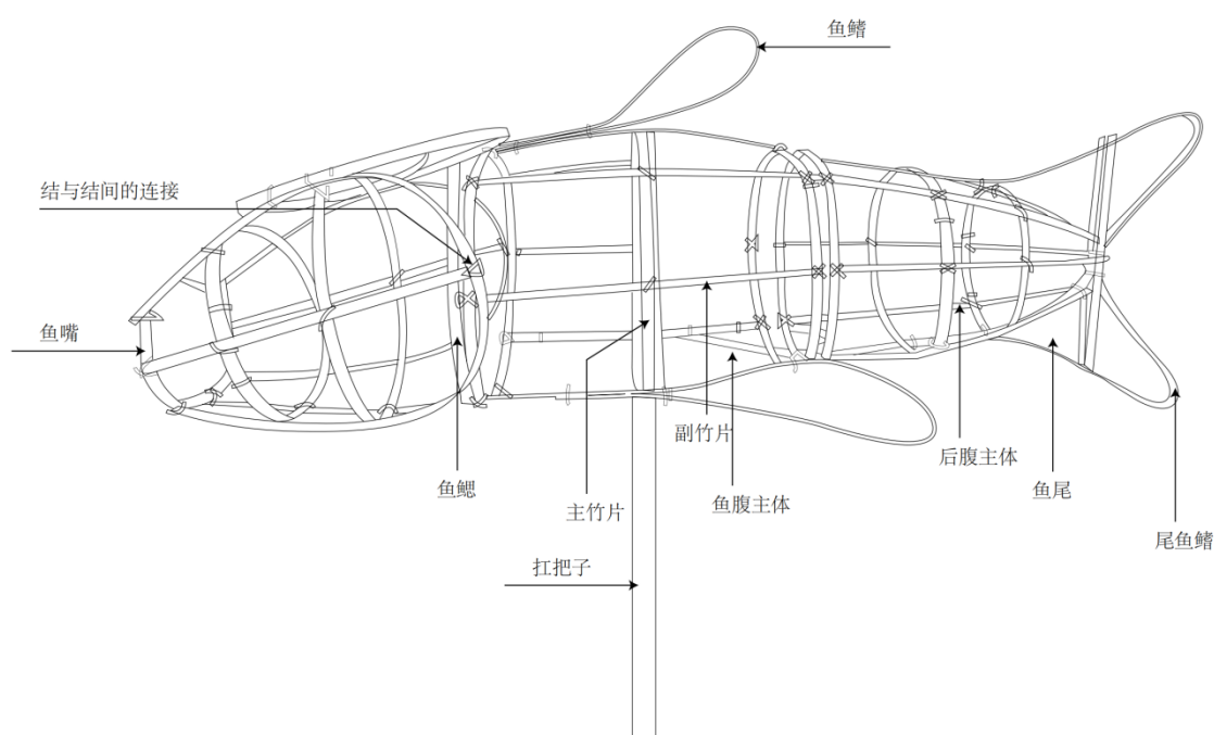
图C.1 渔梁鱼灯骨架示意图
