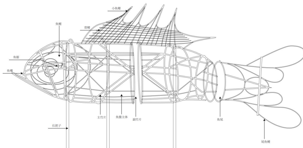
图A.1汪满田鱼灯骨架示意图
